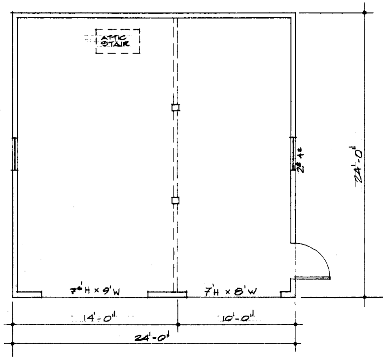
PLAN SCALE: 1/4" = 1'-0"
